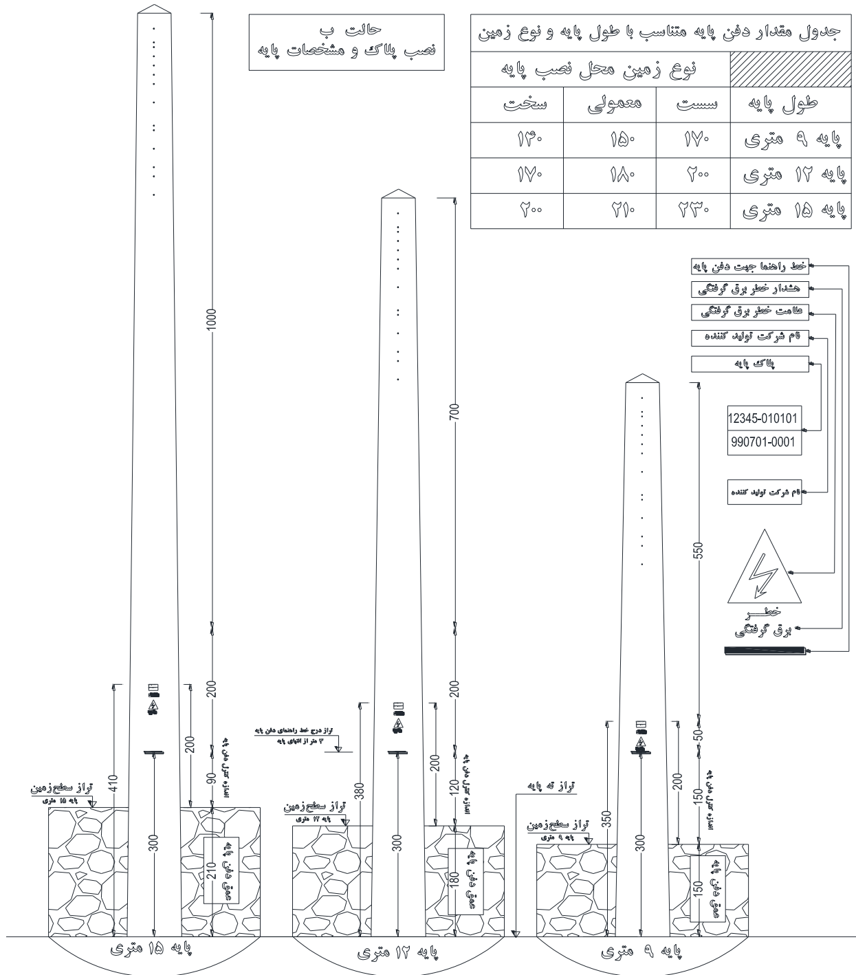
شکل ۱۴- محل درج علائم و نوشتار پایه و موقعیت نوشتار نسبت به عمق مدفون در حالت (ب)
