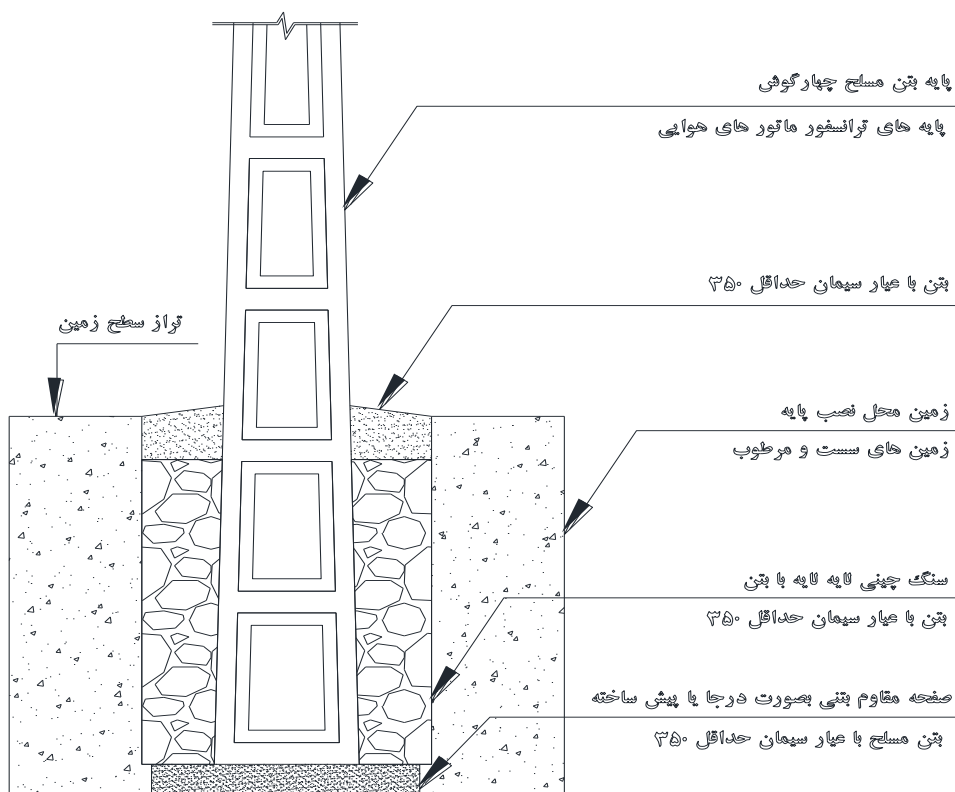
شکل ۱۱- طرح فونداسیون پایه های ترانسفورماتور هوایی در زمین های سست و مرطوب
