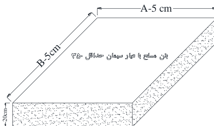
شکل ۴- مشخصات اجرایی بتن فوقانی پایه
